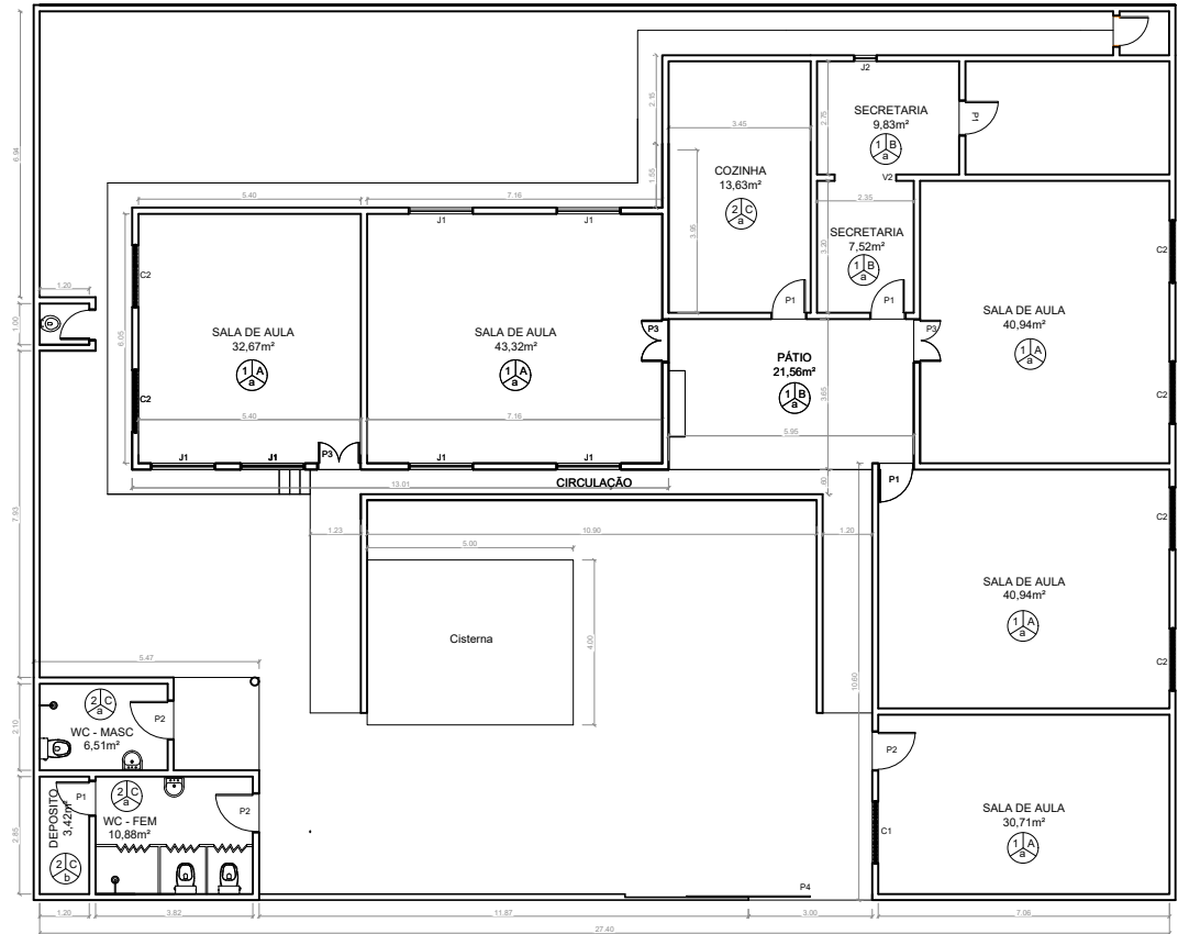
PLANTA BAIXA SITUAÇÃO ATUAL Esc: 1/100
