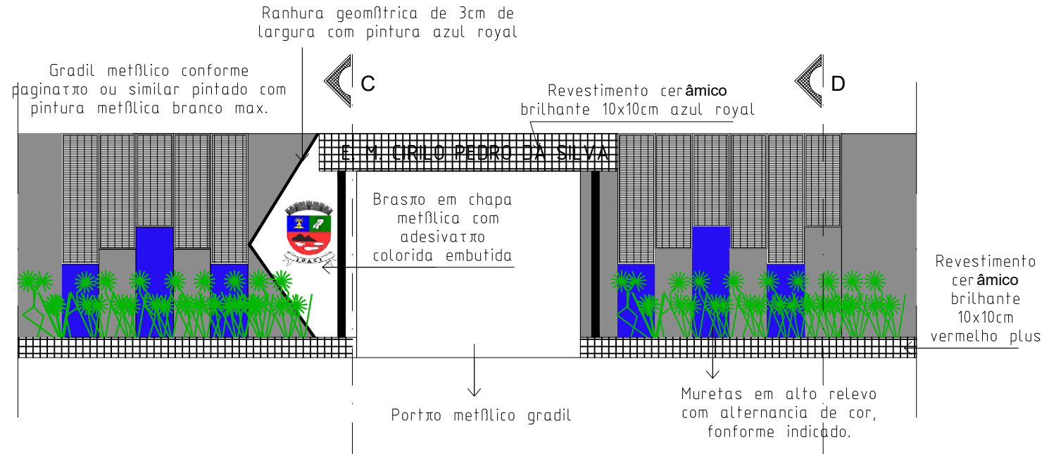
04 FACHADA-MURO Esc: 1/50
