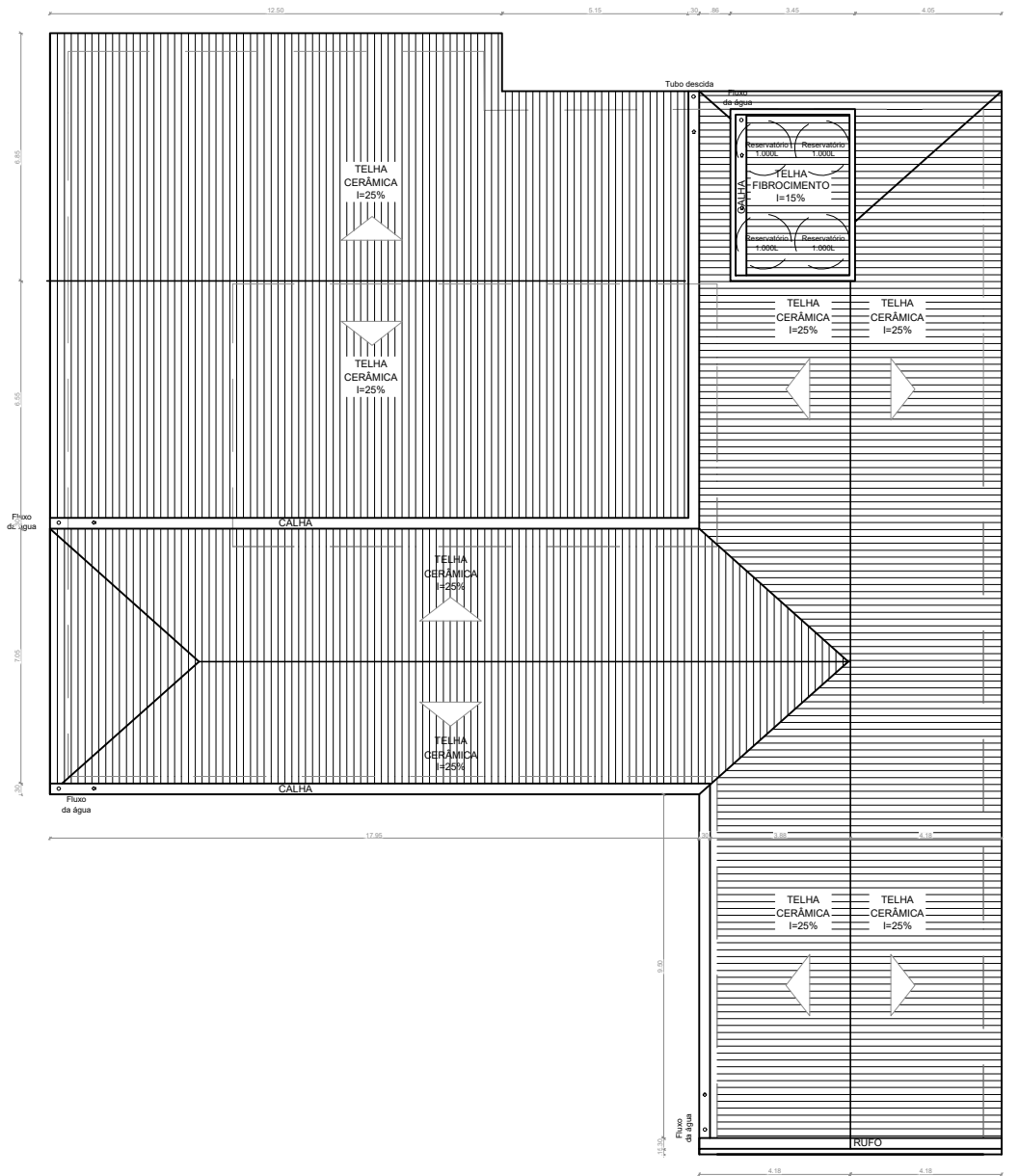
PLANTA DE COBERTURA-LOCAÇÃO Esc. 1/100
