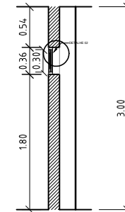
3 J3 CORTE CC' ESCALA 1/25
