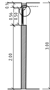
3 J2 CORTE CC' ESCALA 1/25
