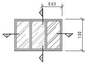
1 VISTA FRONTAL J1 ESCALA 1/25
